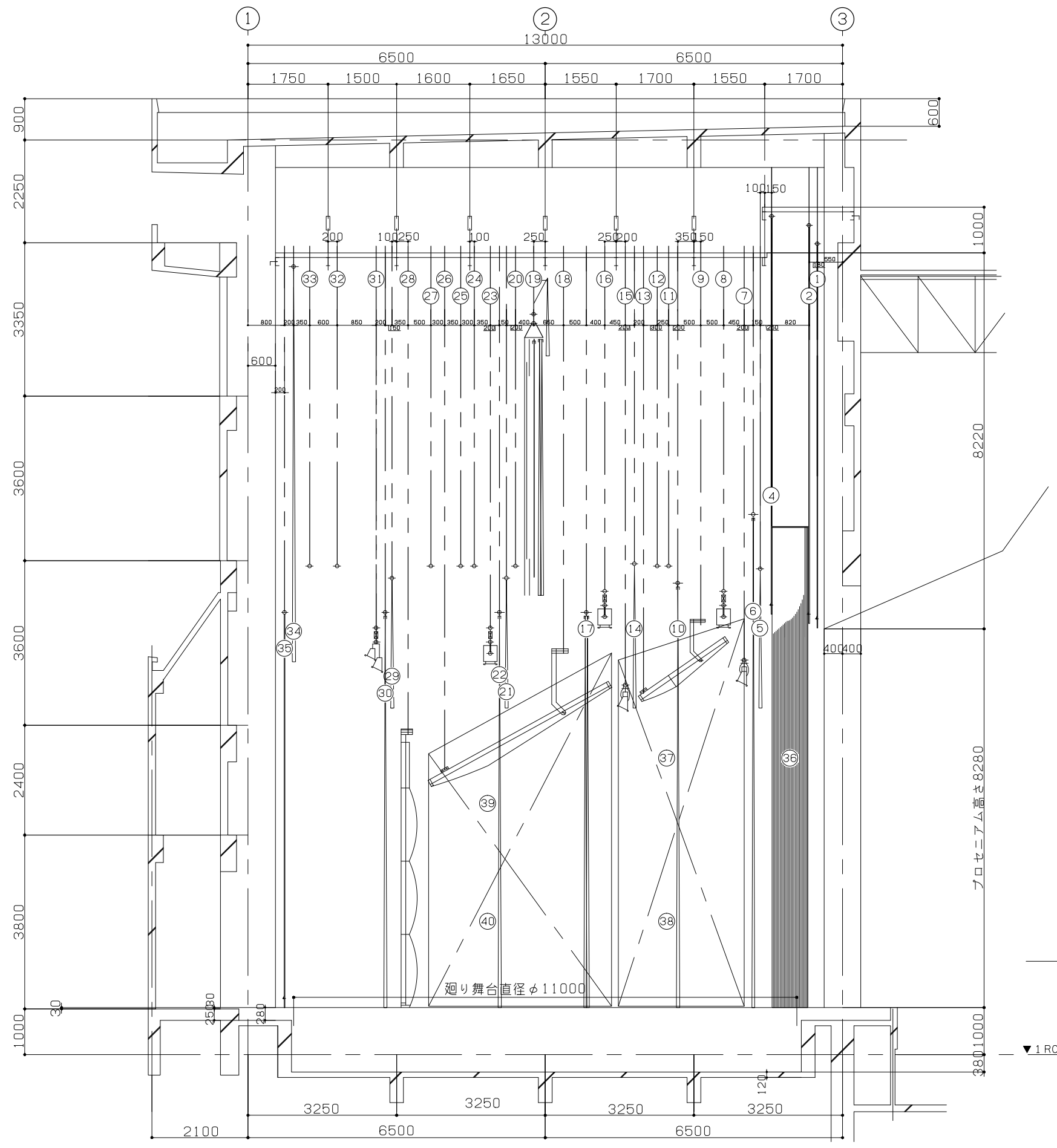
舞台断面図 S=1:100(A3)
